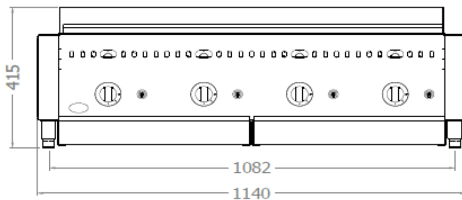
IS 4 Vue de face
