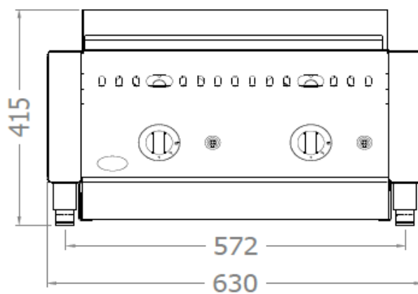
IS 2 Vue de face
