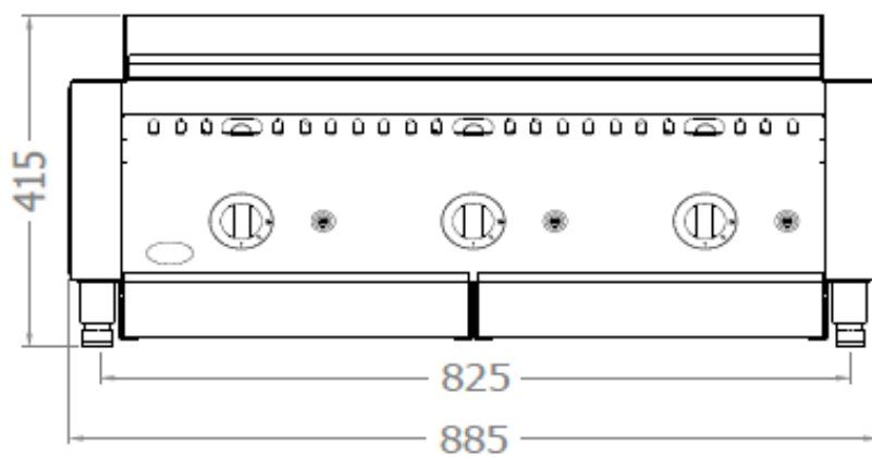
IS 3 Vue de face
