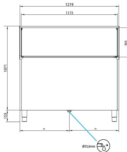
VUE FRONTALE
