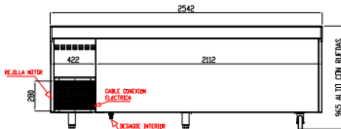
VISTA TRASERA
